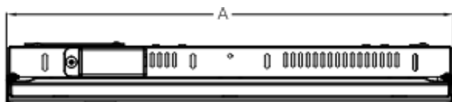
Vista lateral
